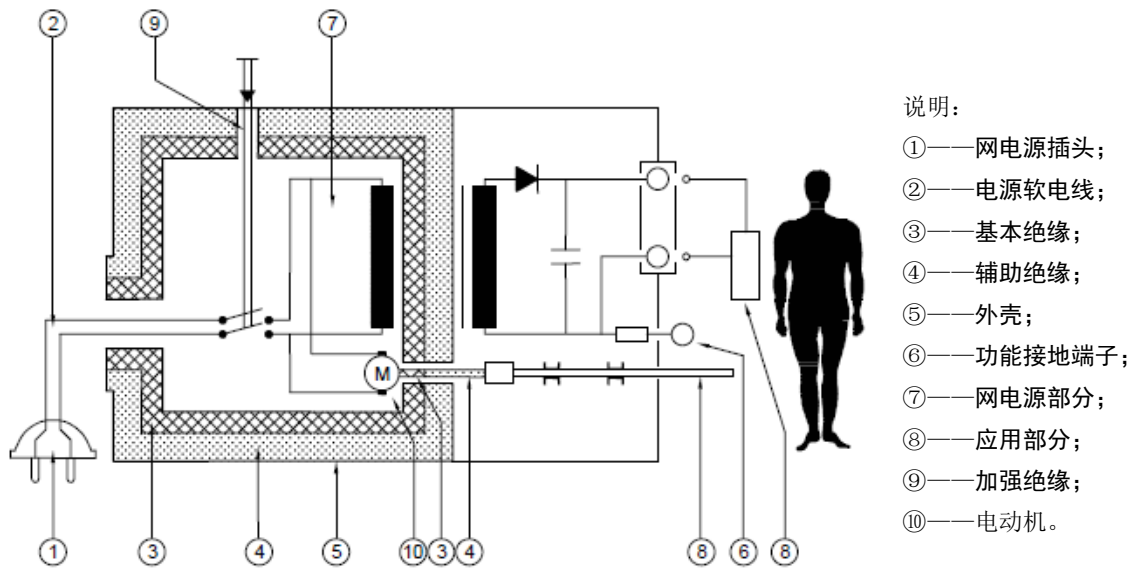
图4 金属包裹的 II 类 ME 设备的示例（见定义）
