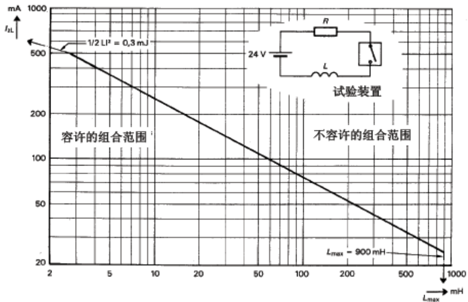
图G.3 在乙醚蒸气和空气混合成的最易燃气体中电感电路上测得的最大容许电流 I_{ZL} 和电感 L_{max} 的函数关系
