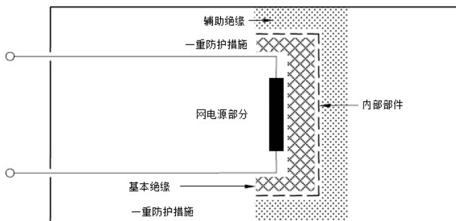
图J.3 绝缘示例 3
