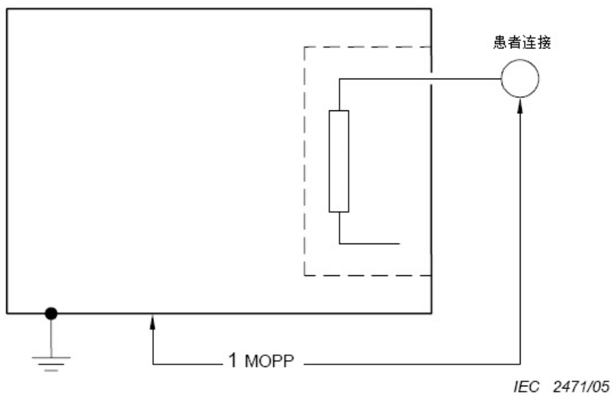
图J.7 绝缘示例 7
