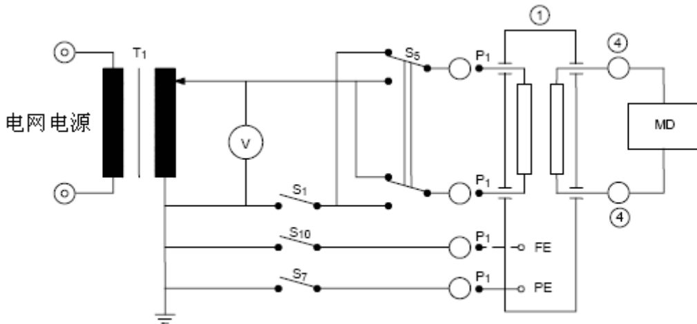
图18 由未保护接地的金属可触及部分上的外来电压引起的从患者连接至地的患者漏电流的测量电路 [见 8. 7. 4. 7d) ]
