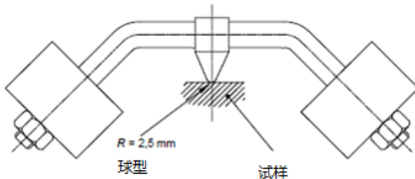
图21 球压试验装置（见 8.8.4.1）
