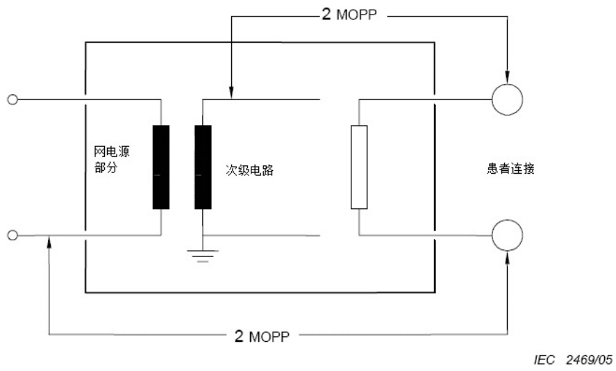
图J.5 绝缘示例 5
