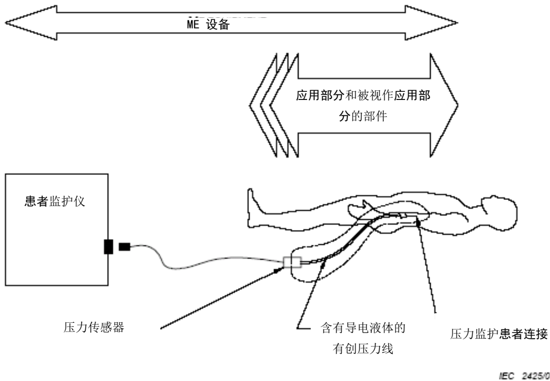
图A.3 附带有创血压监护的病人监护仪中的ME设备，应用部分和患者连接的示例
