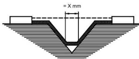
图24 爬电距离和电气间隙——示例 3
