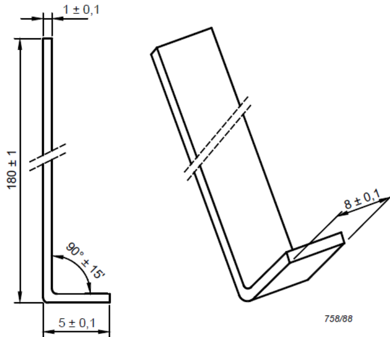
图7 试验钩（见 5.9.2.2）
