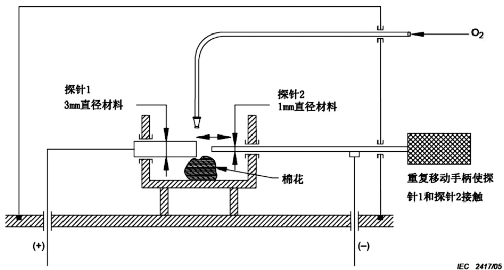
图34 火花点燃试验装置 (见 11. 2. 2. 1)
