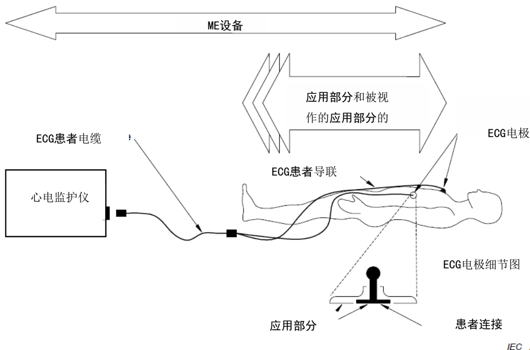
图A.1 心电图监护仪中的 ME 设备，应用部分和患者连接示例
