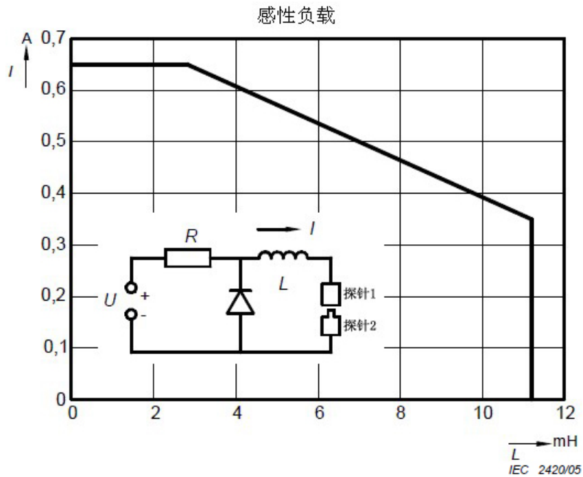
图37 富氧环境感性电路中测得的最大电流 I 和电感 L 的函数关系 (参见 11.2.2.1)
