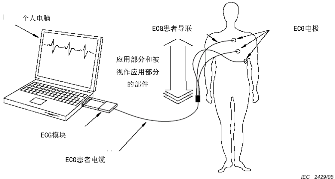
图A.7 有心电模块的个人电脑中的ME设备或ME系统，应用部分和患者连接的示例
