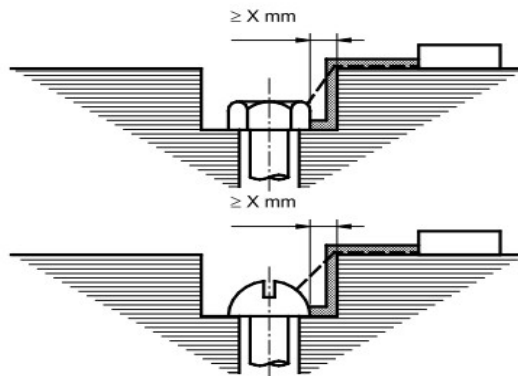
图29 爬电距离和电气间隙——示例 8
