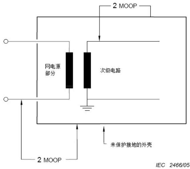
图J.2 绝缘示例 2
