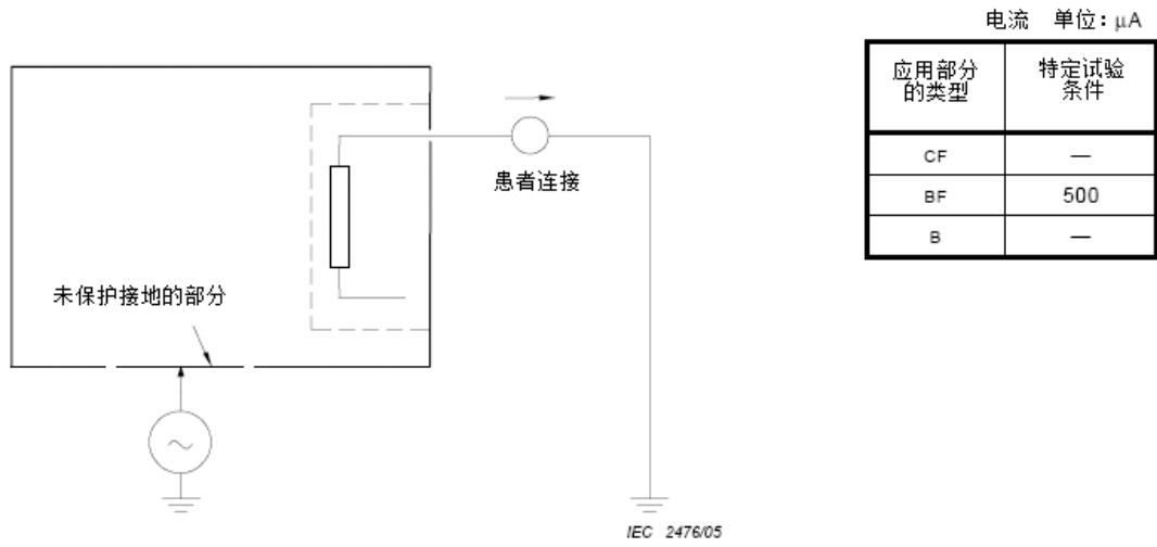
图K. 5 带有 BF 型应用部分患者连接的 ME 设备
