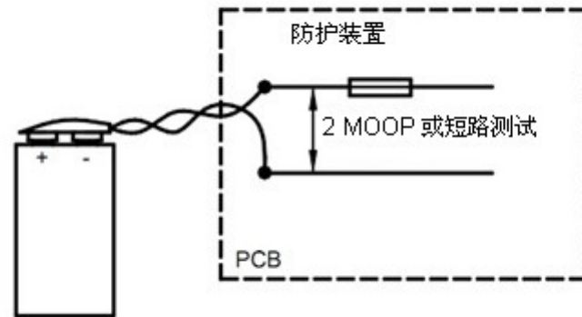
图 A. 23 内部电源端子和随后的防护装置间需要操作者防护措施的示例
