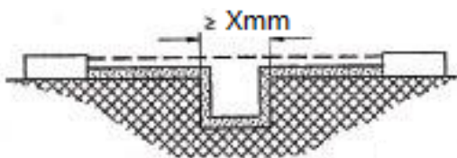
图23 爬电距离和电气间隙——示例 2
