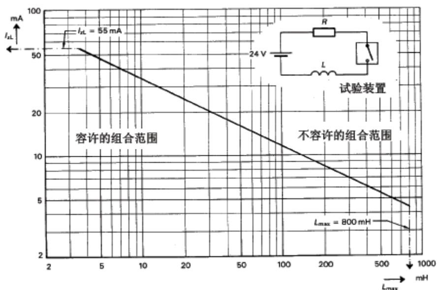
图G.6 在乙醚蒸气和氧混合成的最易燃气体中电感电路上测得的最大容许电流 I_{ZL} 和电感 L_{MAX} 的函数关系
