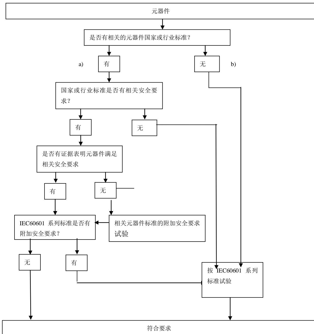
图5 元器件合格性流程图（见 4.8）
