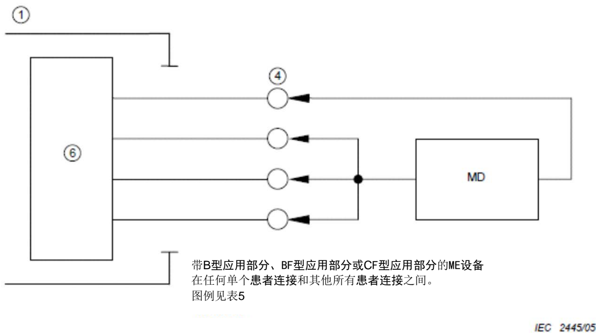
图E.4 患者辅助电流
