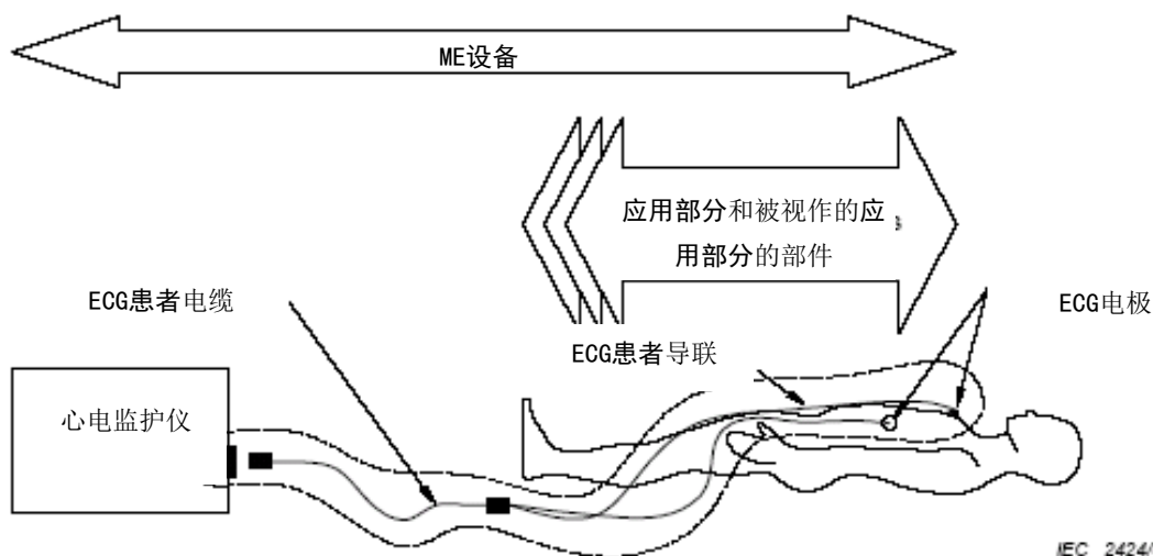
图A.2 在 ME 设备内带绝缘的 F 型应用部分的绝缘示例
