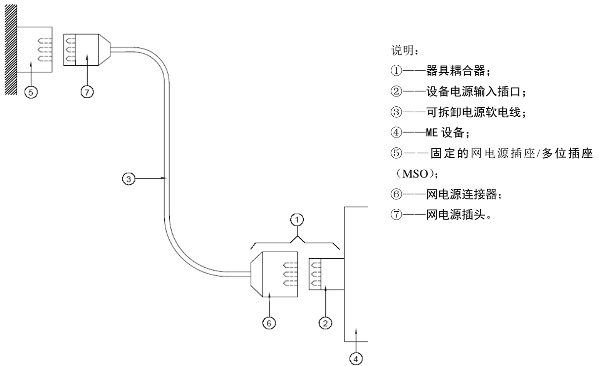
图1 可拆卸的网电源连接（见定义）
