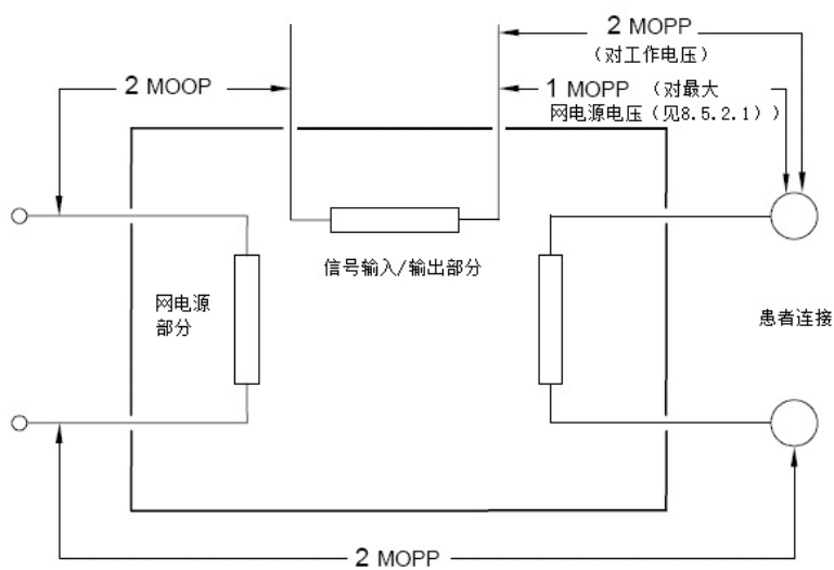
图J.4 绝缘示例 4
