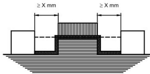
图27 爬电距离和电气间隙——示例 6
