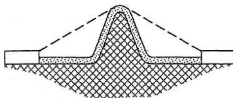
图25 爬电距离和电气间隙——示例 4
