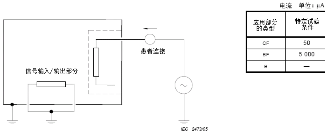
图K. 1 带有由绝缘材料制成的外壳的 ME 设备 (简化的图 15) [见 8. 7. 4. 7a)]
