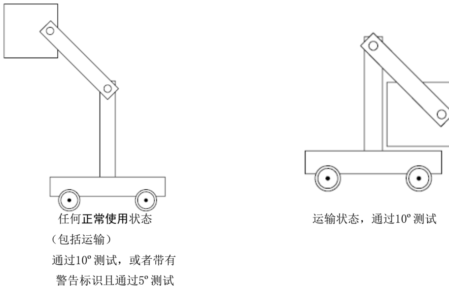
图A.16 不稳定性试验条件
