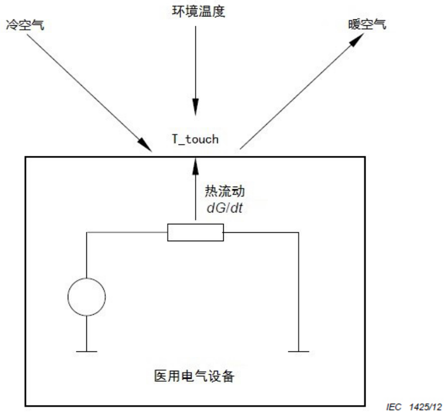
图 A.22 高海拔下设备表面和应用部分的最高容许温度
