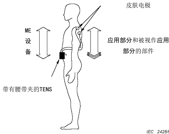
图A.6 由患者佩戴在皮带上且电极连接在患者上臂的经皮电子神经刺激器中 ME 设备,应用部分和患者
