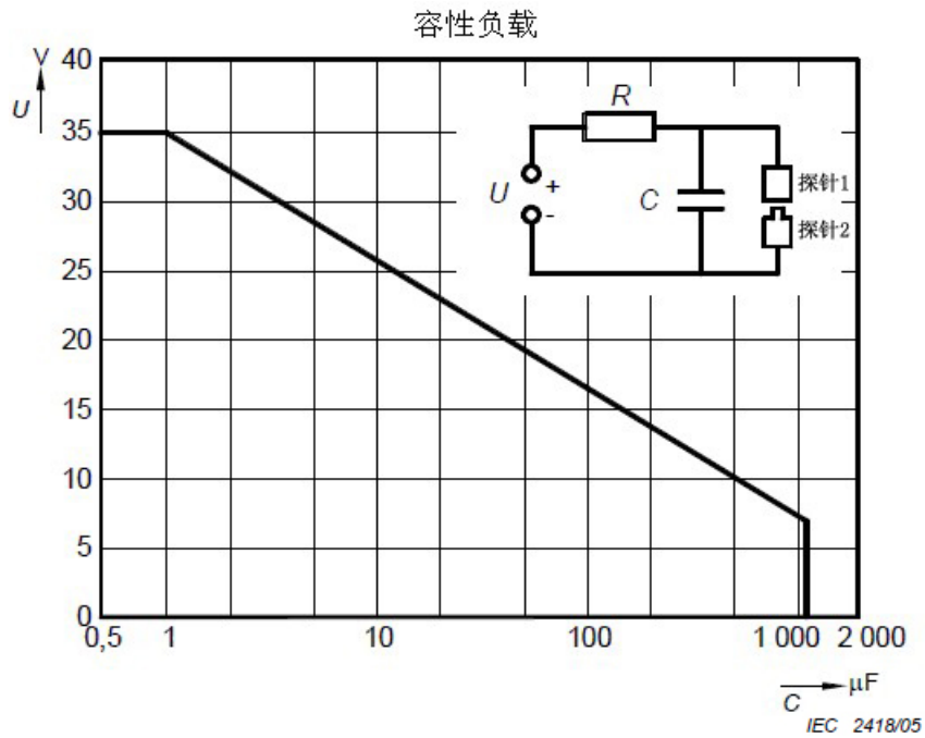
图36 富氧环境容性电路中测得的最大电压 U 和电容 C 的函数关系 (见 11.2.2.1)
