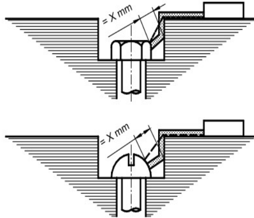
图30 爬电距离和电气间隙——示例 9
