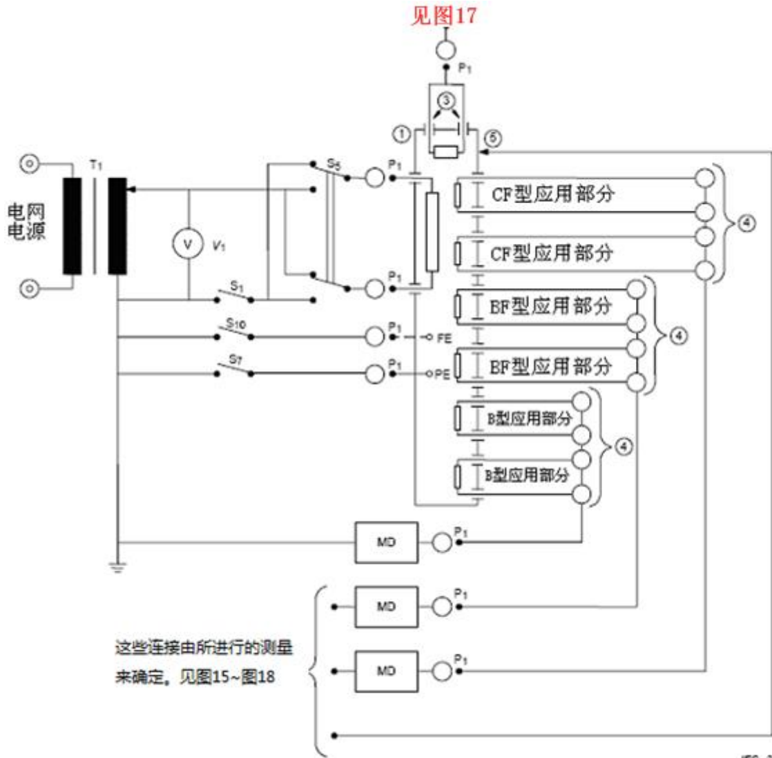
图19 患者辅助电流测量电路（见 8.7.4.8）
