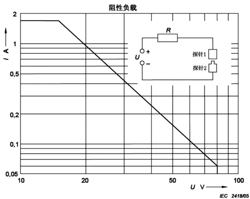
图35 富氧环境纯阻性电路中测得的最大容许电流 I 和最大容许电压 U 的函数关系 (见 11. 2. 2. 1)
