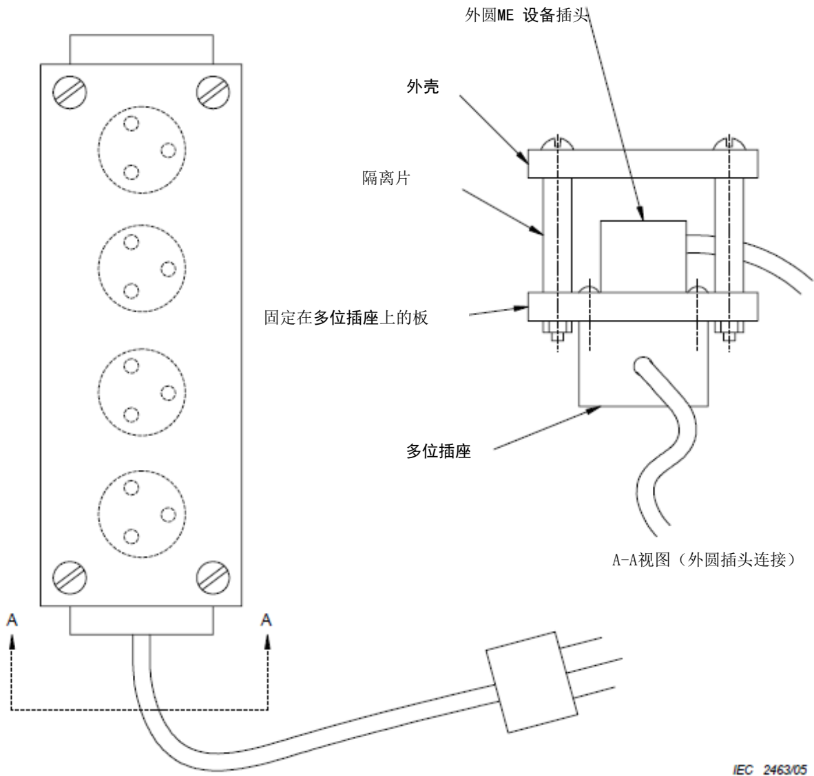
图I.1 多位插座构造的实例 (MSO)
