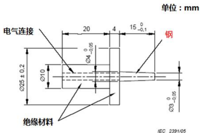
图8 试验针[见 8.4.2d)]
