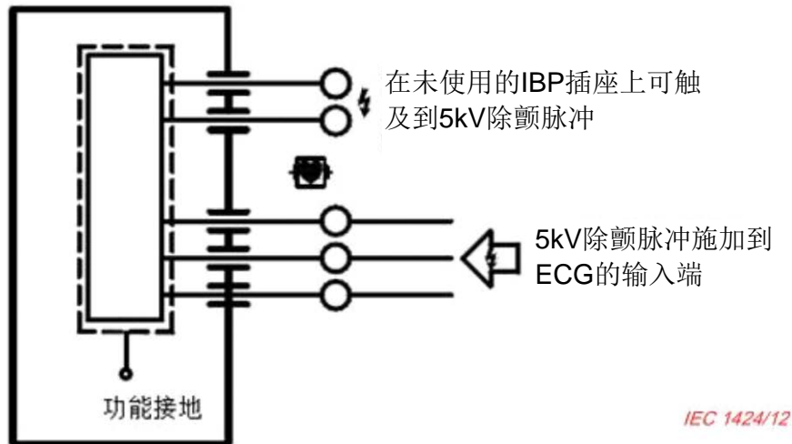
图A. 21 在一个共同的应用部分电路上有两个不同功能的ME设备举例
