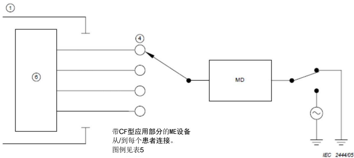
图E.3 CF 型应用部分
