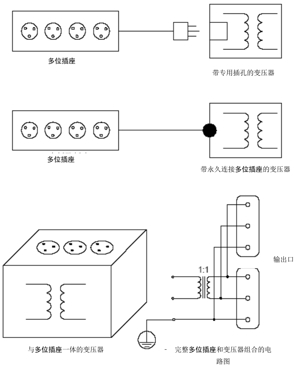
图1.2 多位插座应用的实例
