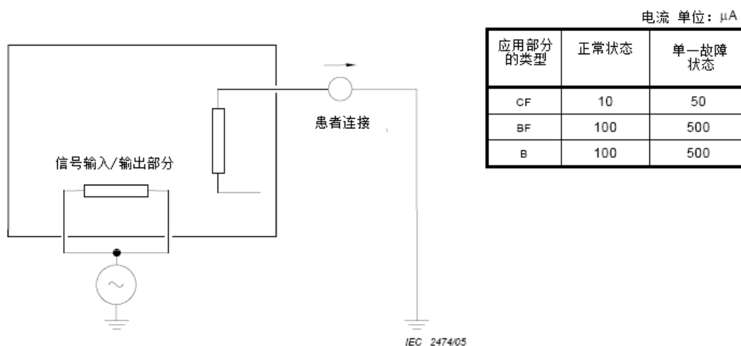
图K. 3 带有应用部分和信号输入/输出部分的 ME 设备
