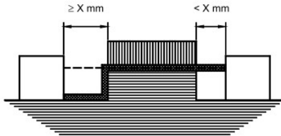
图28 爬电距离和电气间隙——示例 7
