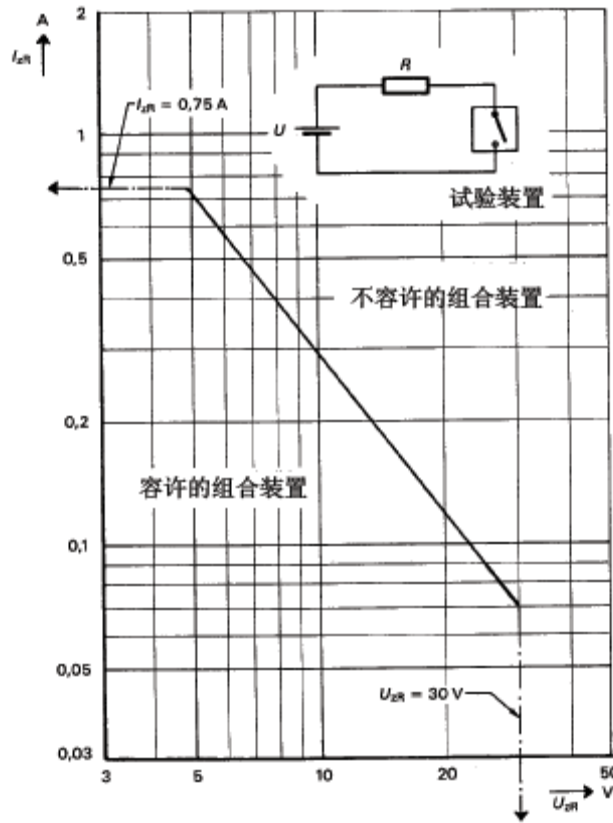
图G.4 乙醚蒸气和氧混合成的最易燃气体中纯电阻电路上测得的最大容许电流 I_{ZR} 和最大容许电压 U_{ZR} 的函数关系
