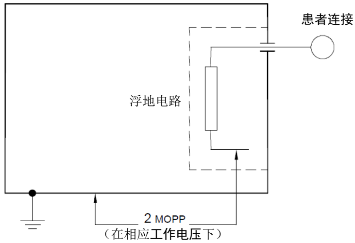
图J.6 绝缘示例 6
