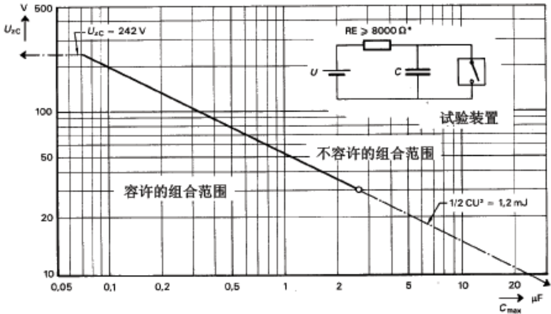
图G.1 在乙醚蒸气和空气混合成的最易燃气体中纯电阻电路上测得的最大容许电流 I_{ZR} 和最大容许电压 U_{ZR} 的函数关系
