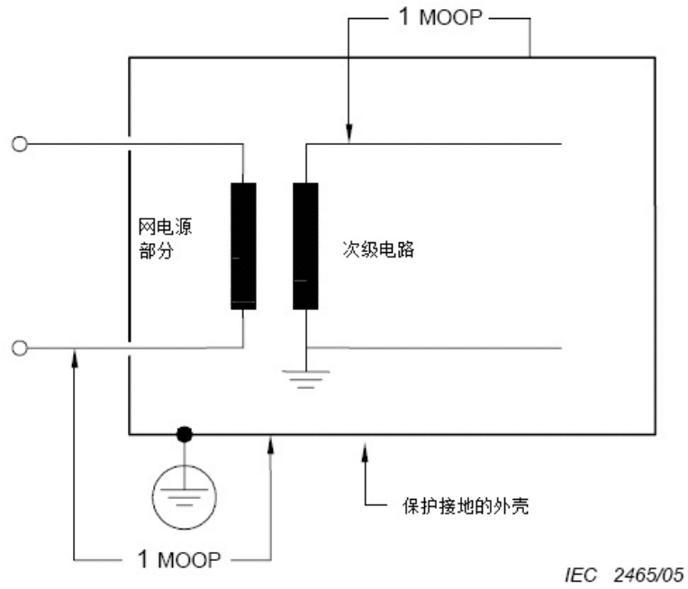
图J.1 绝缘示例 1
