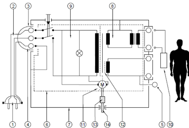
图3 I 类 ME 设备的示例 (见定义)
